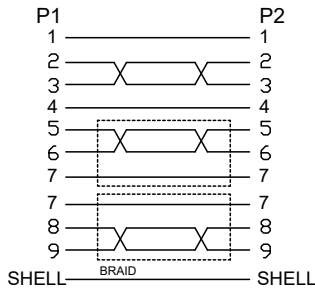
Anschlussdiagramm / Wiring diagram
